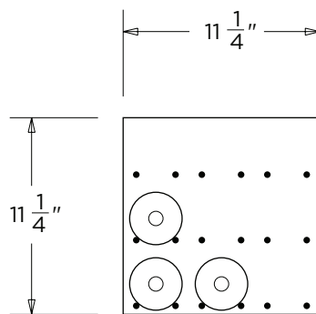
3,3 Module shown
